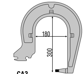
CA3 ARM + ELECTRODE L=300 mm - ● 803171
